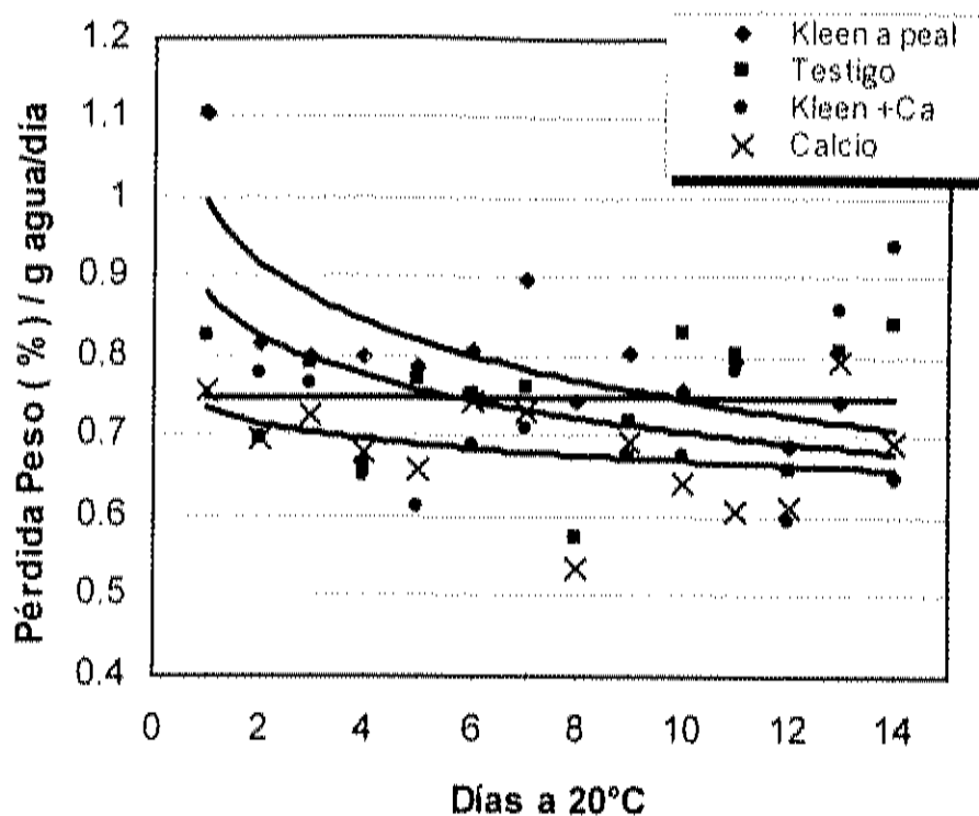
Figura 5. Transpiración diaria normalizada en frutos de chile bell pepper tratados con ácidos carboxílicos y calcio almacenados a 20°C. Las líneas representan la tendencia de cada uno de los tratamientos.
