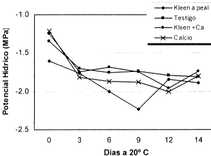
Figura 8. Potencial Hídrico en frutos de chile bell pepper tratados con ácidos carboxílicos y calcio almacenados a 20°C
