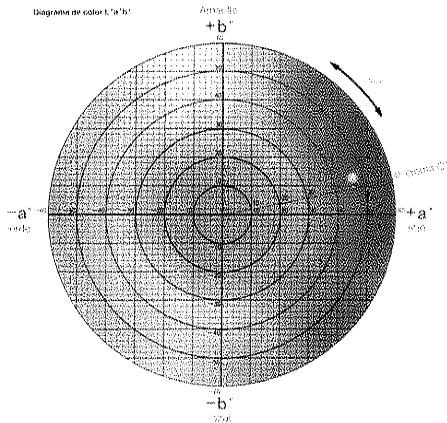
Figura 2. Círculo de color que expresa la cromaticidad o dirección del color por medio de las coordenadas a^* y b^* .
